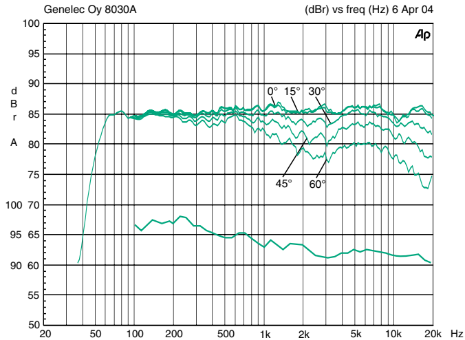
Illustration 5. Le groupe de courbes montre les caractéristiques de directivité horizontale de la 8030A mesurées à 1 m. La courbe inférieure montre la réponse en puissance de l'enceinte.
