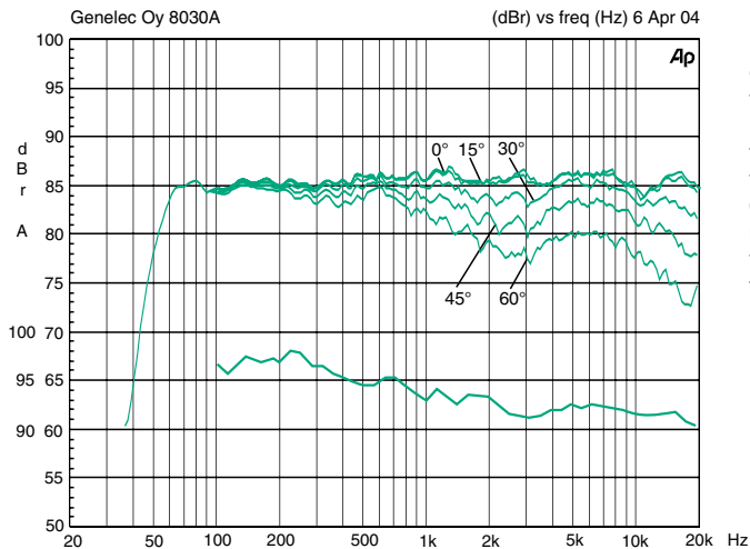
Figur 5. Den övre gruppen av kurvor visar den horisontella riktningsskarakteristiken hos 8030A mätt vid 0, 15, 30, 45 samt 60 graders vinkel på 1 m avstånd. Den undre visar systemets effektkurva
