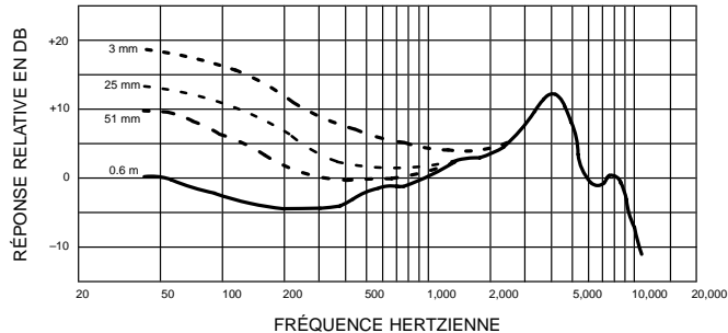
COURBE DE RÉPONSE TYPIQUE FIGURE 1
