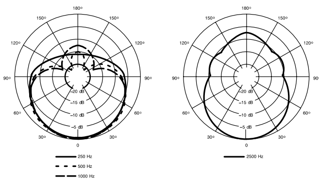
TYPISCHE POLARCHARAKTERISTIK ABBILDUNG 2
